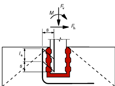
Cimentación en el caso del pilar con claves.
