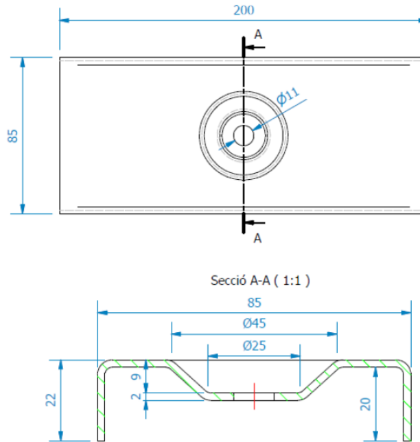
Figura 4.1 Cotas generales BIG-80
