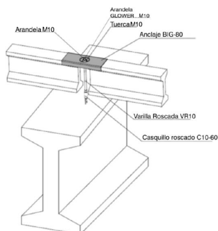
Figura 2.1 Sistema ensamblado
