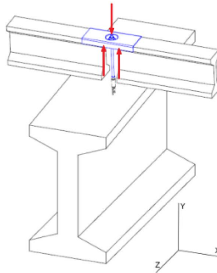
Figura 6.1 Esquema de acciones sobre el BIG-80
