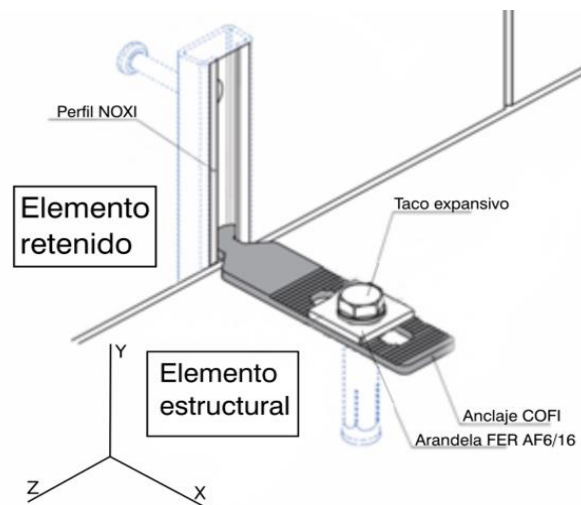
Figura 2.2 Montaje COFI con un perfil
