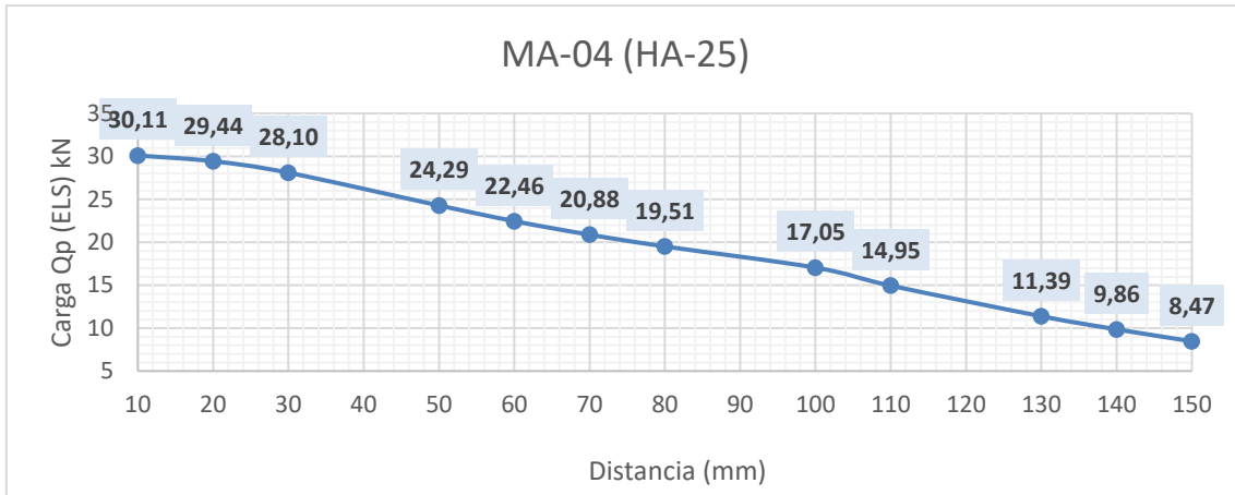
Gráfico 6.7 Cargas máximas (Qp) en función del voladizo
