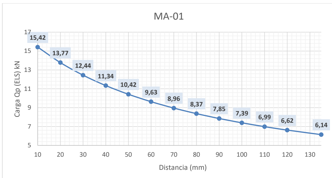
Gráfico 6.61 Cargas máximas (Qp) en función del voladizo
