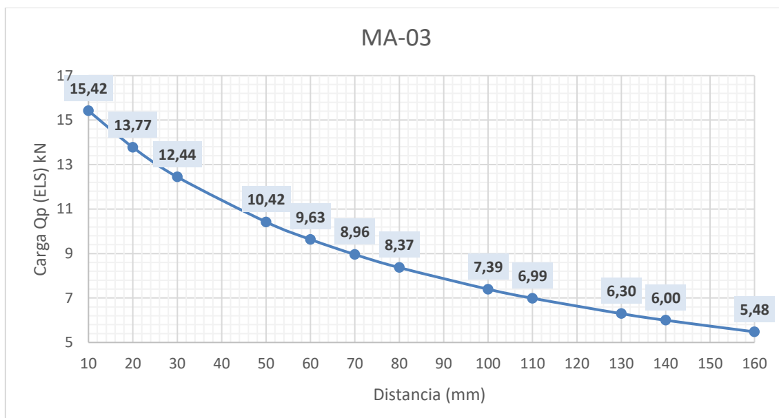
Gráfico 6.63 Cargas máximas (Qp) en función del voladizo
