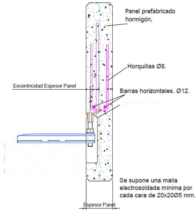
Figura 8.5 Vista lateral de la armadura adicional
