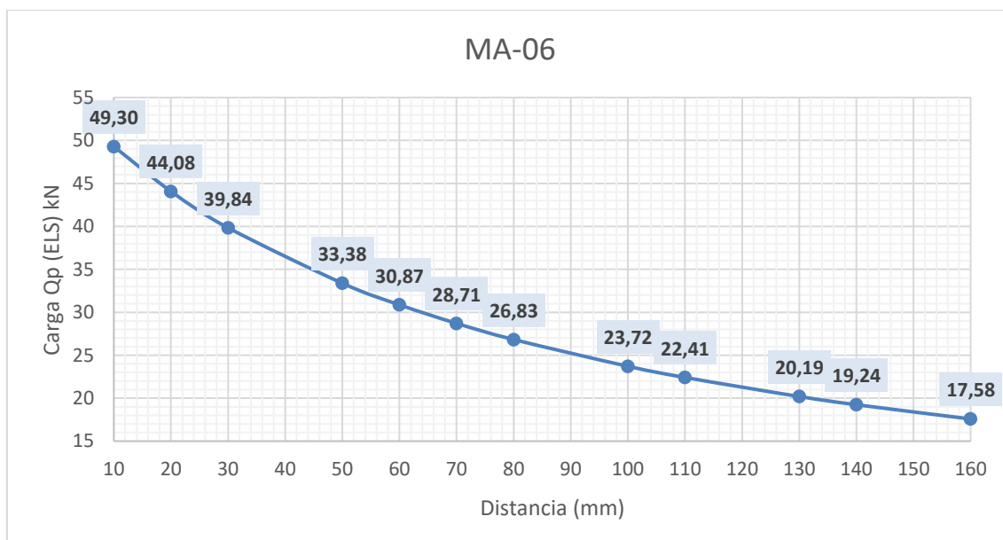
Gráfico 6.66 Cargas máximas (Qp) en función del voladizo
