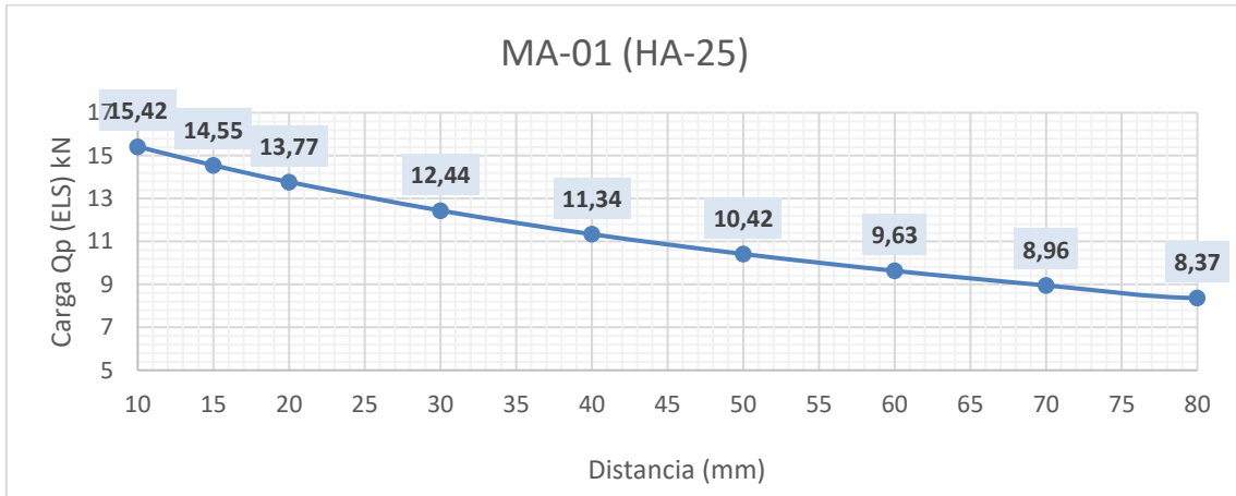
Gráfico 6.1 Cargas máximas (Qp) en función del voladizo
