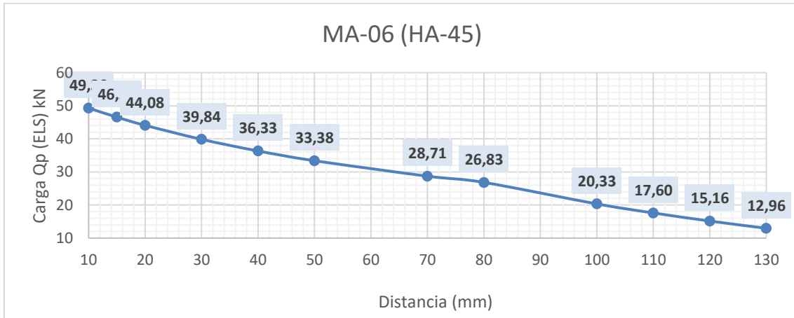
Gráfico 6.59 Cargas máximas (Qp) en función del voladizo
