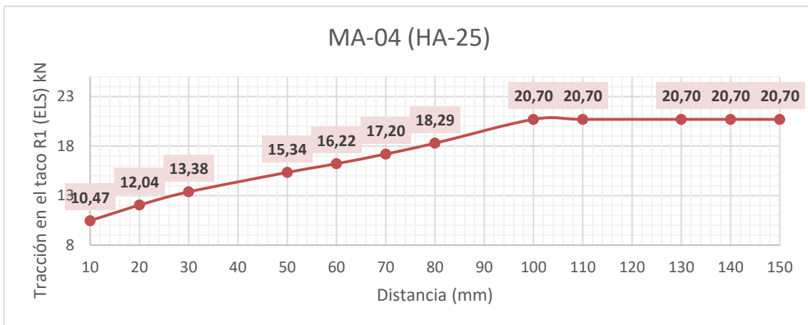
Gráfico 6.8 Reacciones (R1) en función del voladizo
