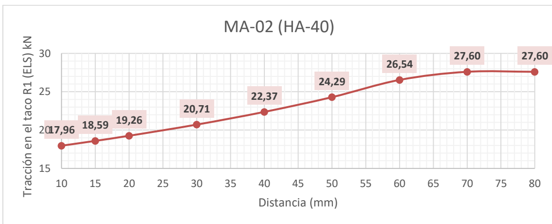
Gráfico 6.40 Reacciones (R1) en función del voladizo
