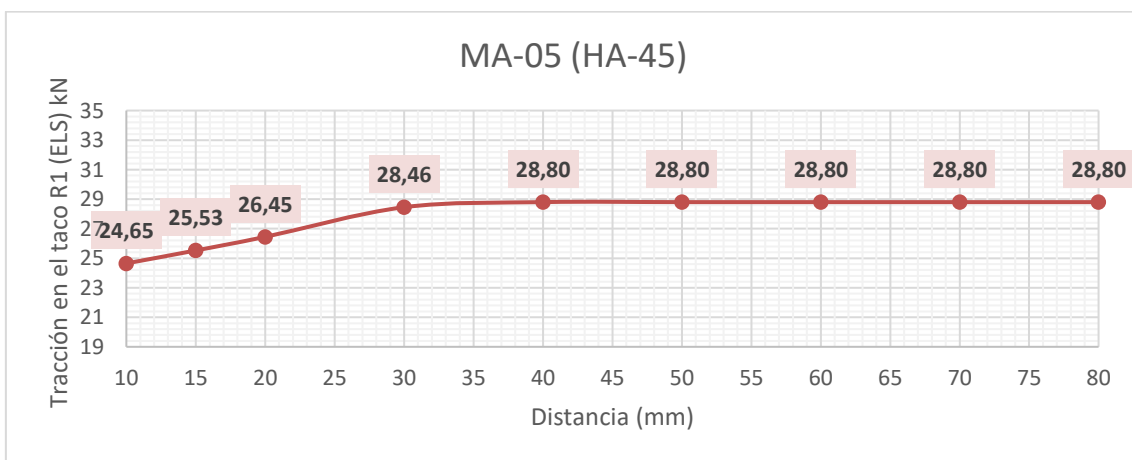
Gráfico 6.58 Reacciones (R1) en función del voladizo
