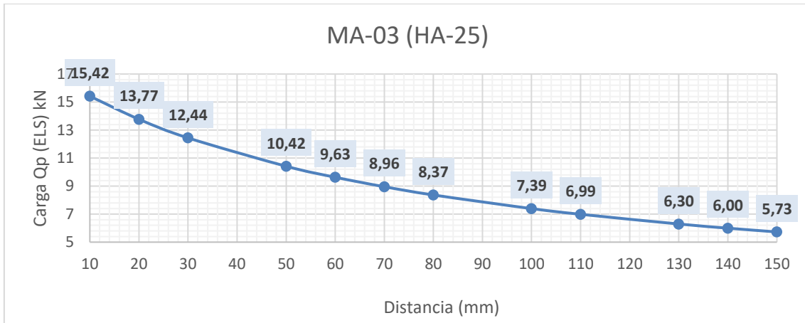
Gráfico 6.5 Cargas máximas (Qp) en función del voladizo
