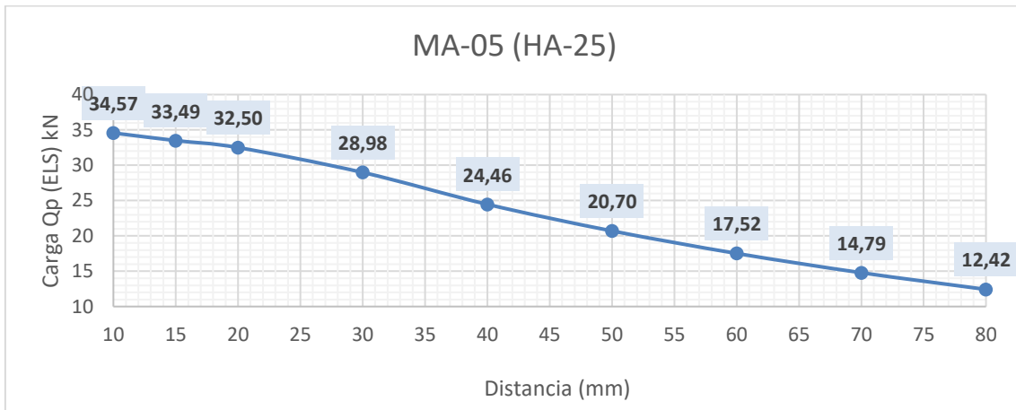
Gráfico 6.9 Cargas máximas (Qp) en función del voladizo
