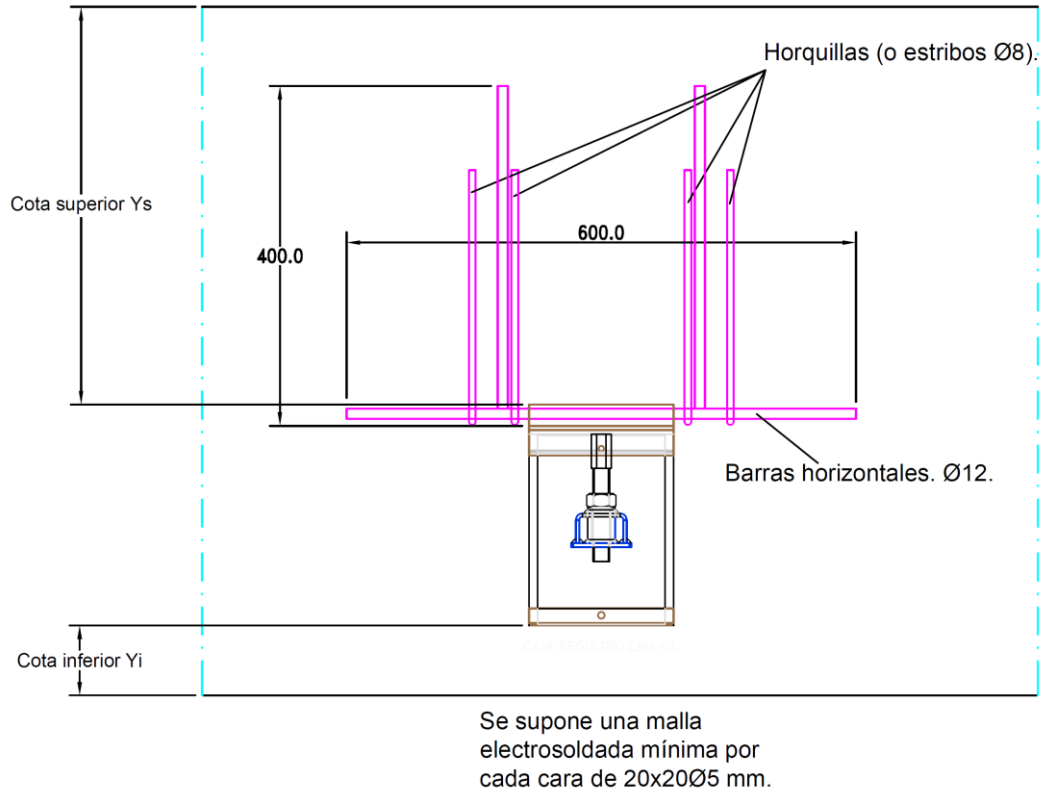
Figura 8.4 Disposición de armadura adicional para la CMA
