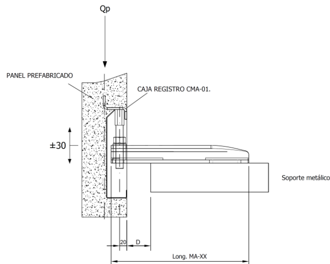
Figura 6.1 MA sobre soporte metálico
