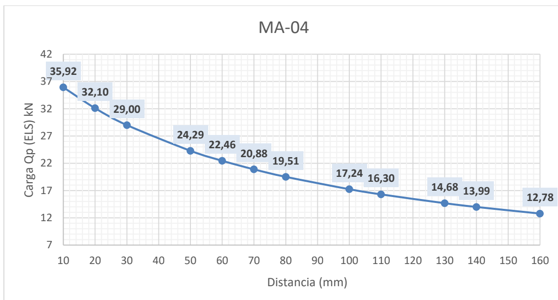
Gráfico 6.64 Cargas máximas (Qp) en función del voladizo
