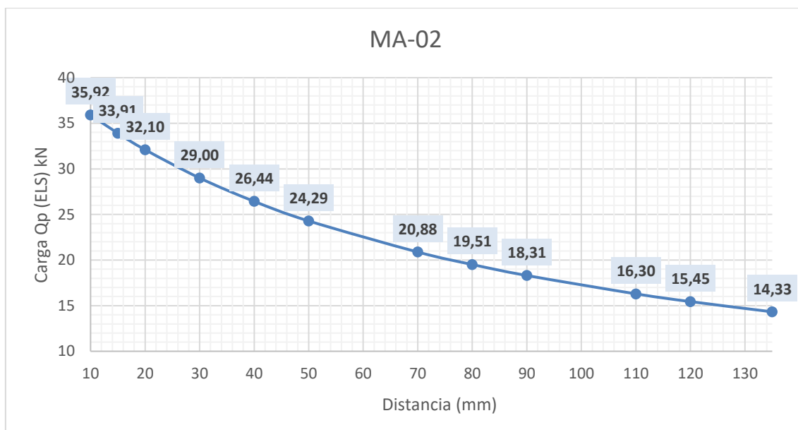
Gráfico 6.62 Cargas máximas (Qp) en función del voladizo
