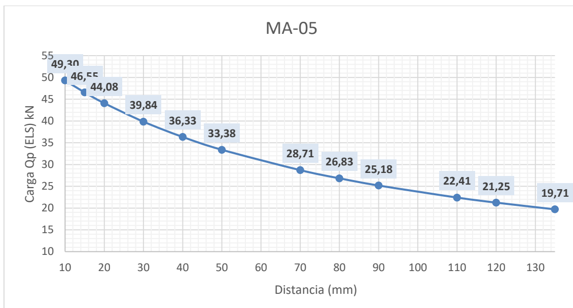
Gráfico 6.65 Cargas máximas (Qp) en función del voladizo
