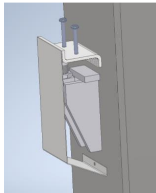
Figura 7.3 Montaje de la ménsula MI-SOL con caja CMI-02-120
