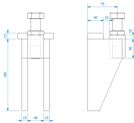
Figura 3.1 Dimensiones MI-SOL
