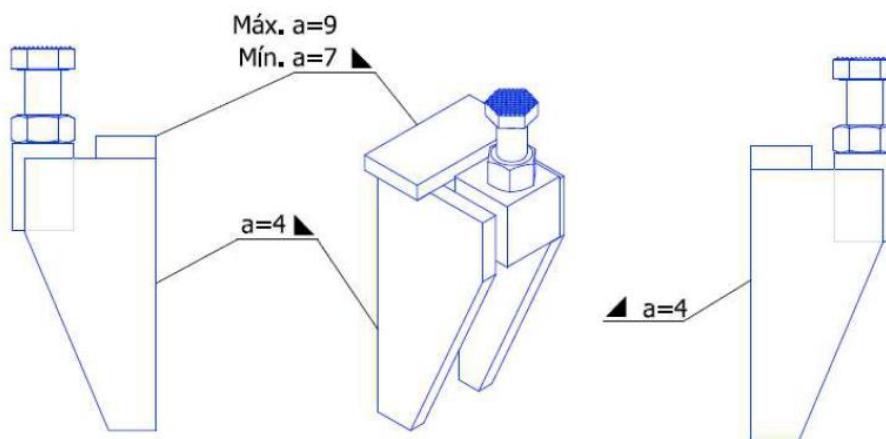
Figura 5.1 Esquema de soldaduras en obra
