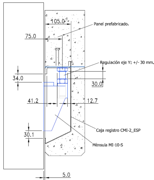
Figura 2.1 Esquema de montaje final de la ménsula MI-SOL y la caja CMI-02
