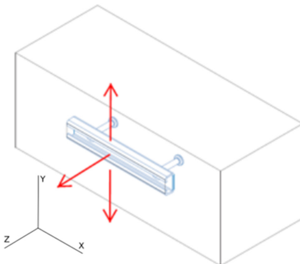
Figura 6.1 Esquema de aplicación de fuerzas
