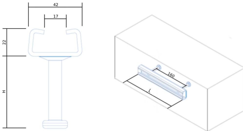
Figura 5.1 Dimensiones del perfil NOXI R
