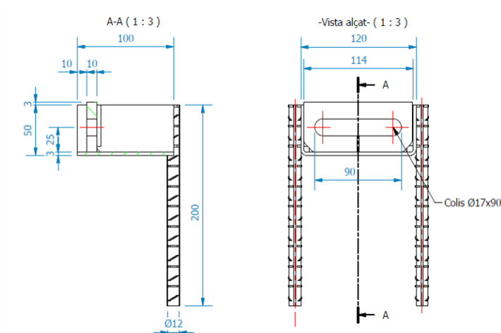
Figura 5.1 Dimensiones OCULFIX 10
