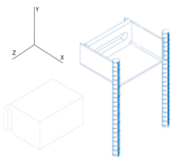
Figura 2.1 Esquema OCULFIX 10
