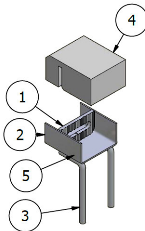
Figura 2.1 Vista explotada del OCULFIX 30
