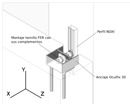
Figura 2.2 OCULFIX 30 ensamblado en el panel
