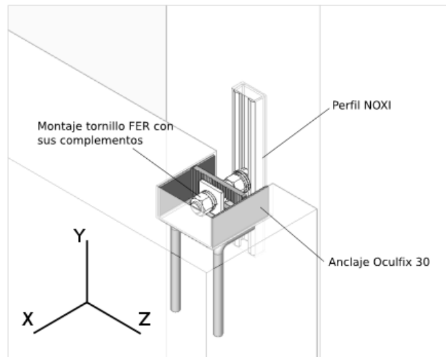
Figura 8.1 Esquema de regulaciones
