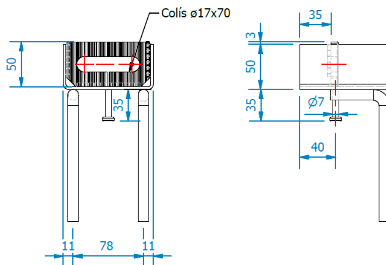
Figura 5.1 Dimensiones OCULFIX 30
