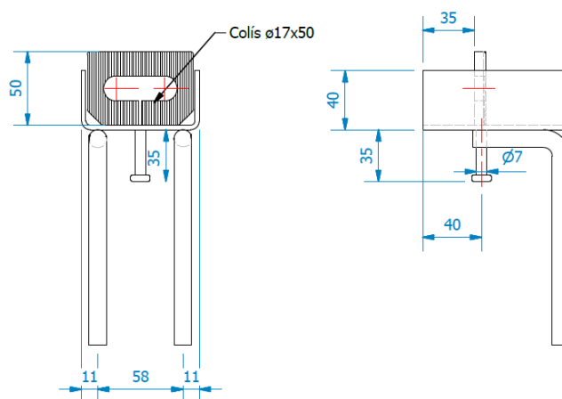
Figura 5.1 Dimensiones OCULFIX 40
