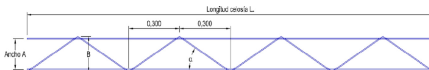
Figura 3.1 Cotas generales de la celosía CEL
