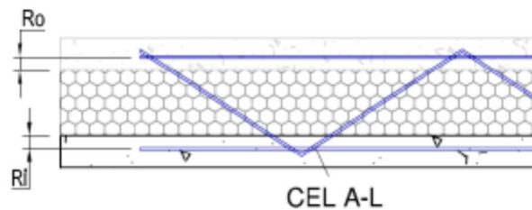
Figura 6.1 Cotas de anclaje mínimas CEL
