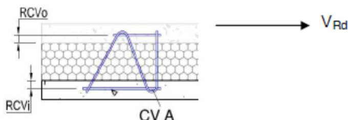
Figura 6.3 Cotas de anclaje mínimas conector viga
