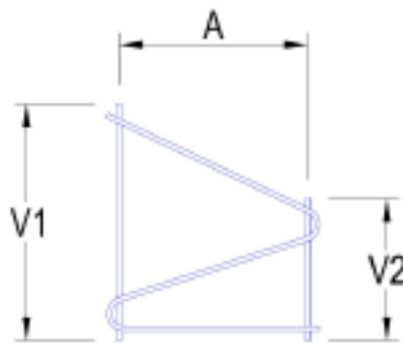
Figura 3.3 Cotas generales del conector viga
