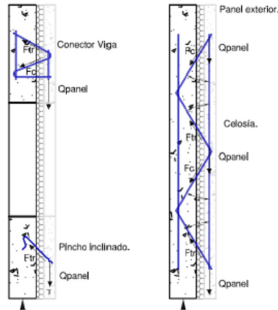
Figura 7.2 Esquema de cargas de peso propio sobre el panel
