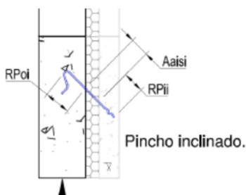
Figura 10.6 Conector PIN colocado de forma inclinada
