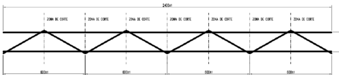
Figura 10.1 Zonas de corte de las celosías CEL
