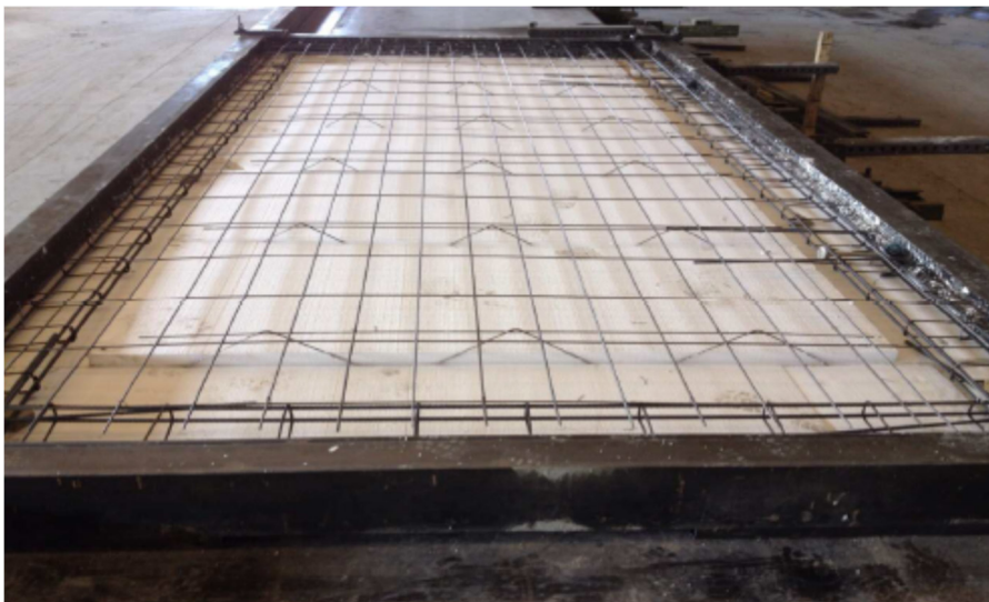
Figura 9.1 Celosías colocadas en panel horizontal sin puente térmico
