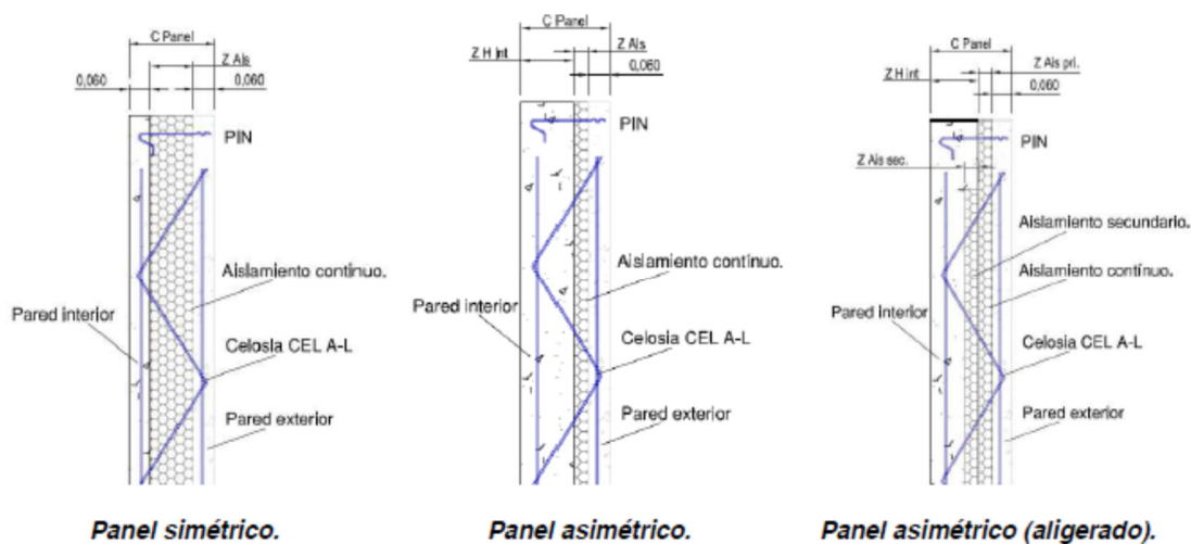
Figura 10.3 Disposición de celosías i conectores según el tipo de panel
