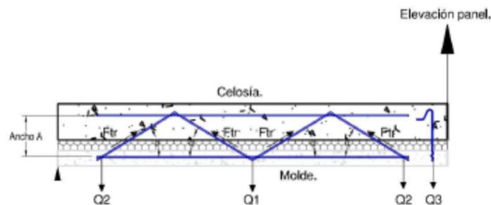
Figura 7.1 Esquema de carga externa aplicada sobre el panel
