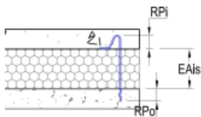
Figura 6.2 Cotas de anclaje mínimas PIN
