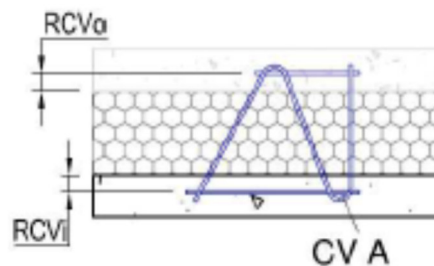
Figura 10.7 Cotas de anclaje mínimas conector viga
