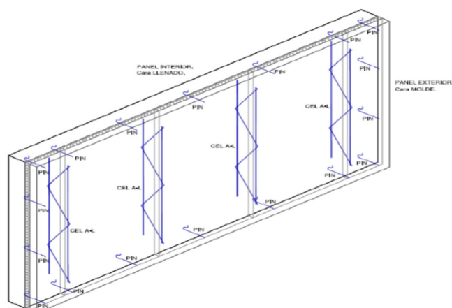
Figura 2.1 Distribución de celosías CEL en un panel
