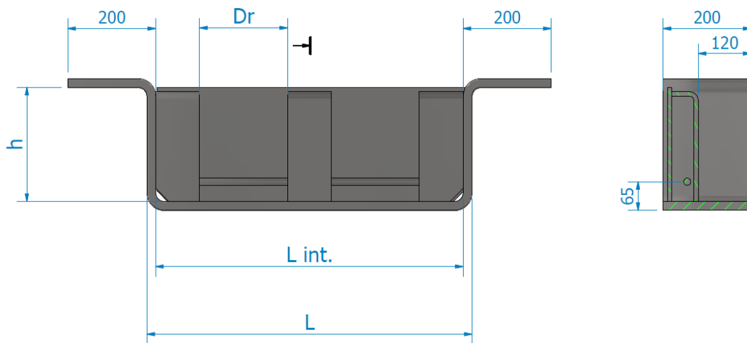
Figura 5.1 Cotas generales de la SOPRA
