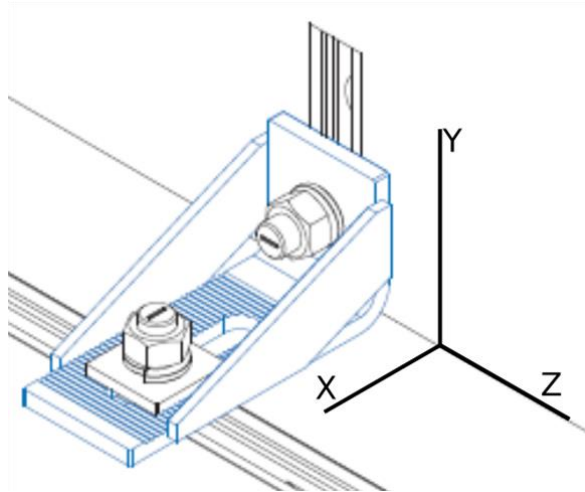
Figura 8.1 Ejes de regulación
