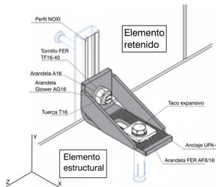
Figura 2.2 Montaje UPA-C con un perfil NOXI
