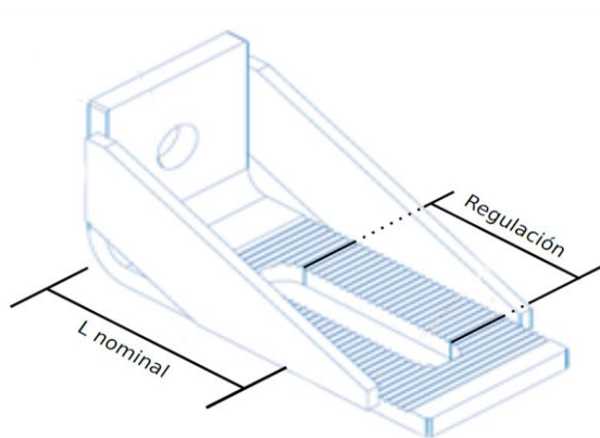
Figura 5.1 Dimensiones UPA-C
